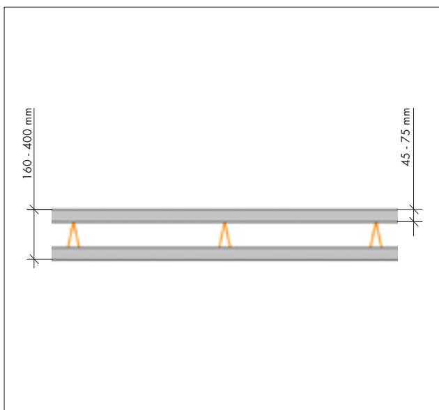
Horisontell sektion skalvägg
