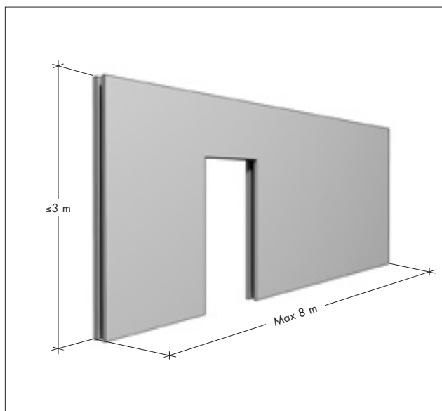
Väggelevation stående transport
