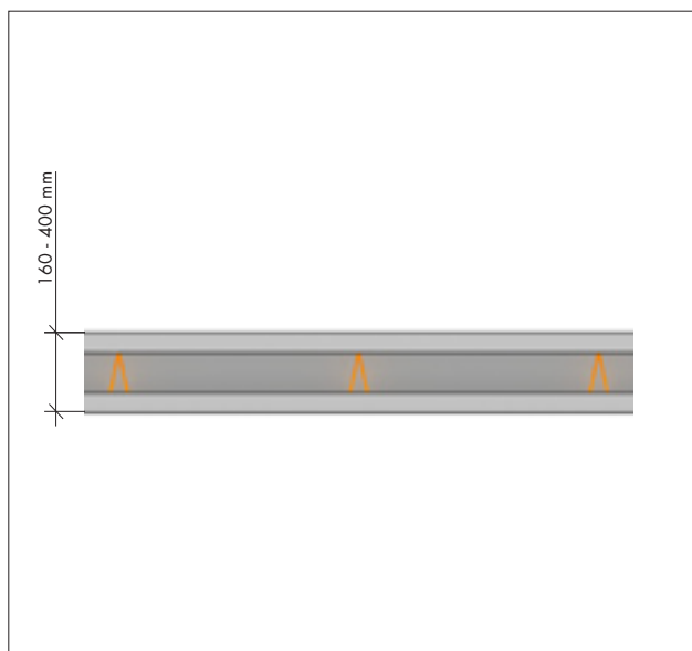
Horisontell sektion massivvägg
