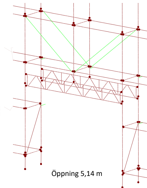
Ställning med överbrygningsbalk enligt punkt 1. Extra väggfästen är placerade på 2,5 m höjd vid sidan om öppningen. I övrigt väggfästen enligt punkt 3.
