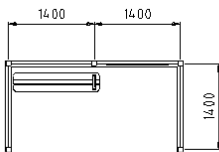
2-SEKTIONER
