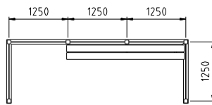
3-SEKTIONER
